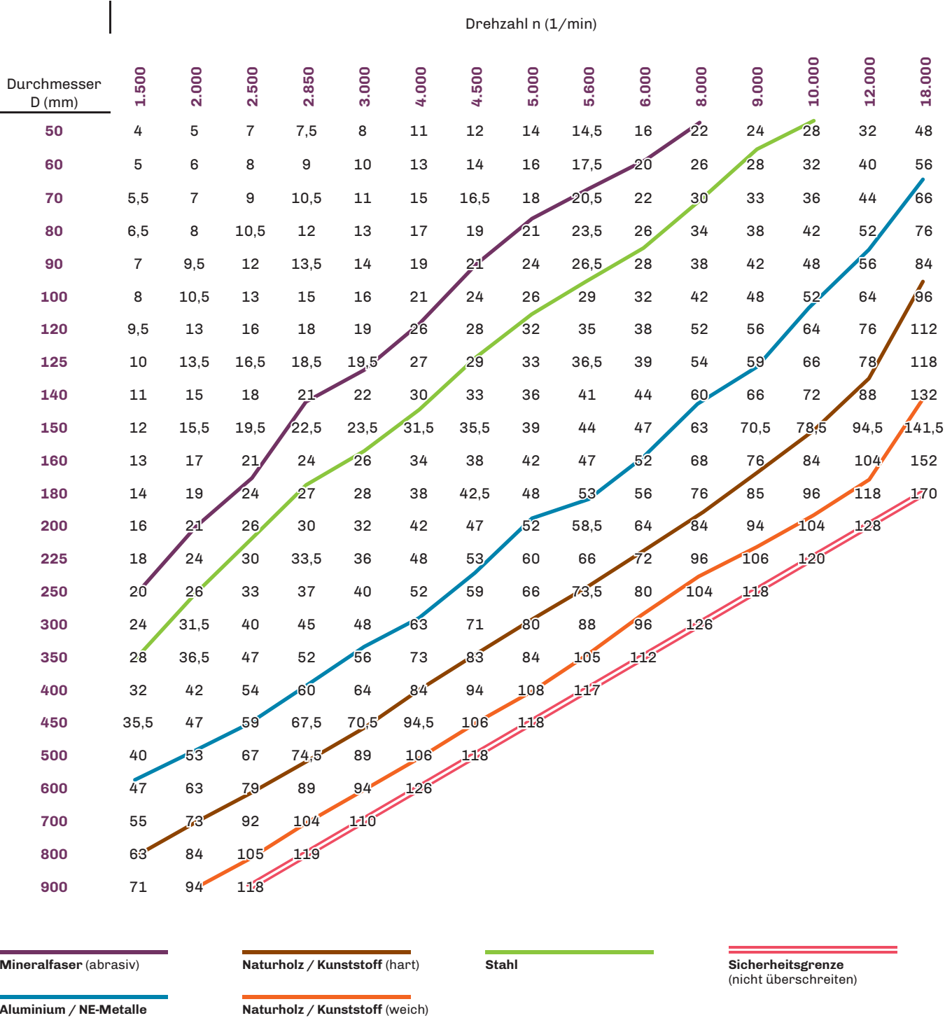
Schnittgeschwindigkeitsdiagramm für Kreissägeblätter zur Bearbeitung abrasiver Materialien
