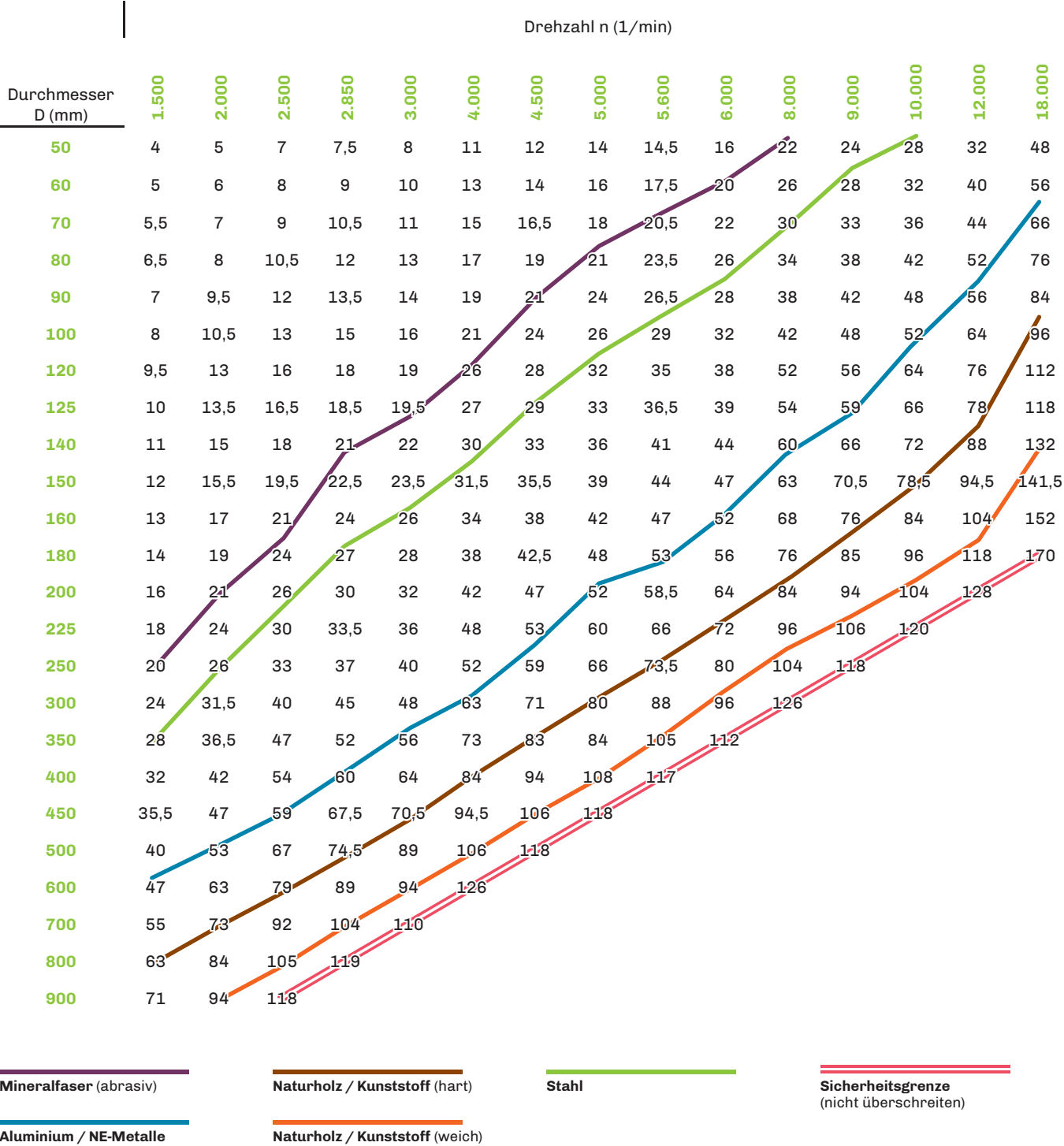
Schnittgeschwindigkeitsdiagramm für Kreissägeblätter im Bereich Bau
