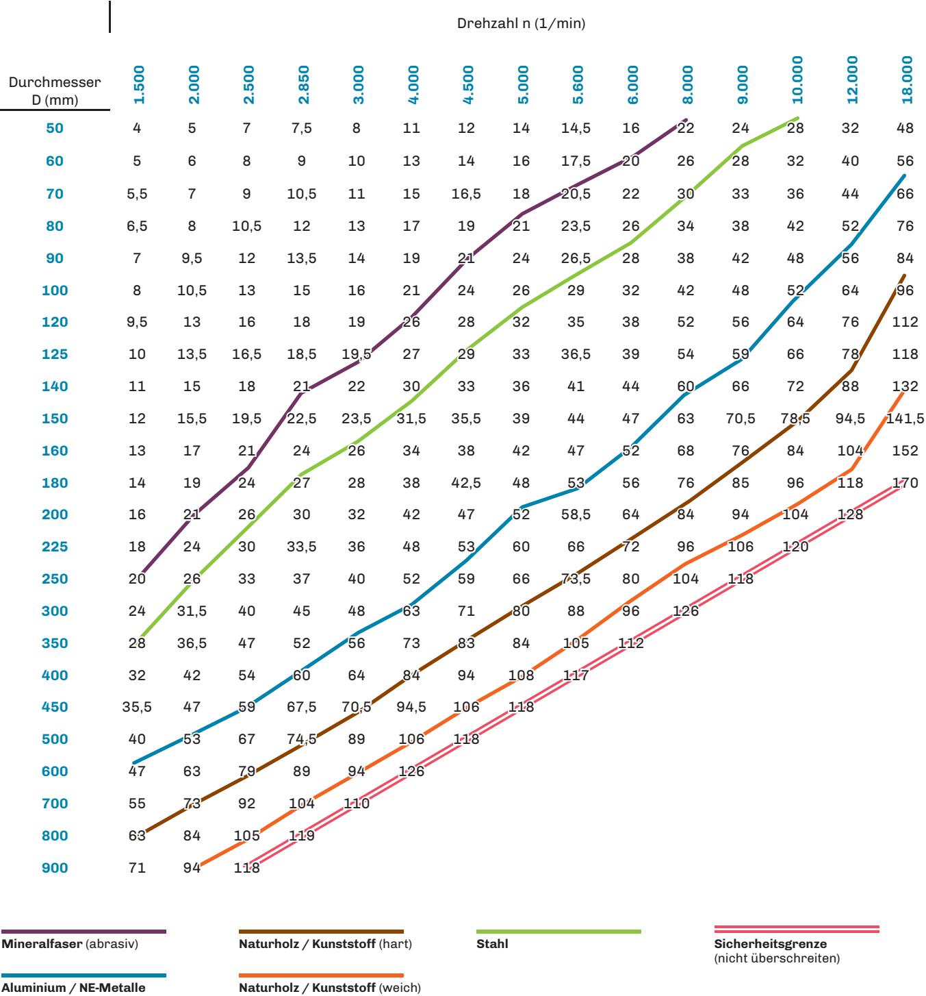
Schnittgeschwindigkeitsdiagramm für Kreissägeblätter zur Bearbeitung von NE-Metallen
